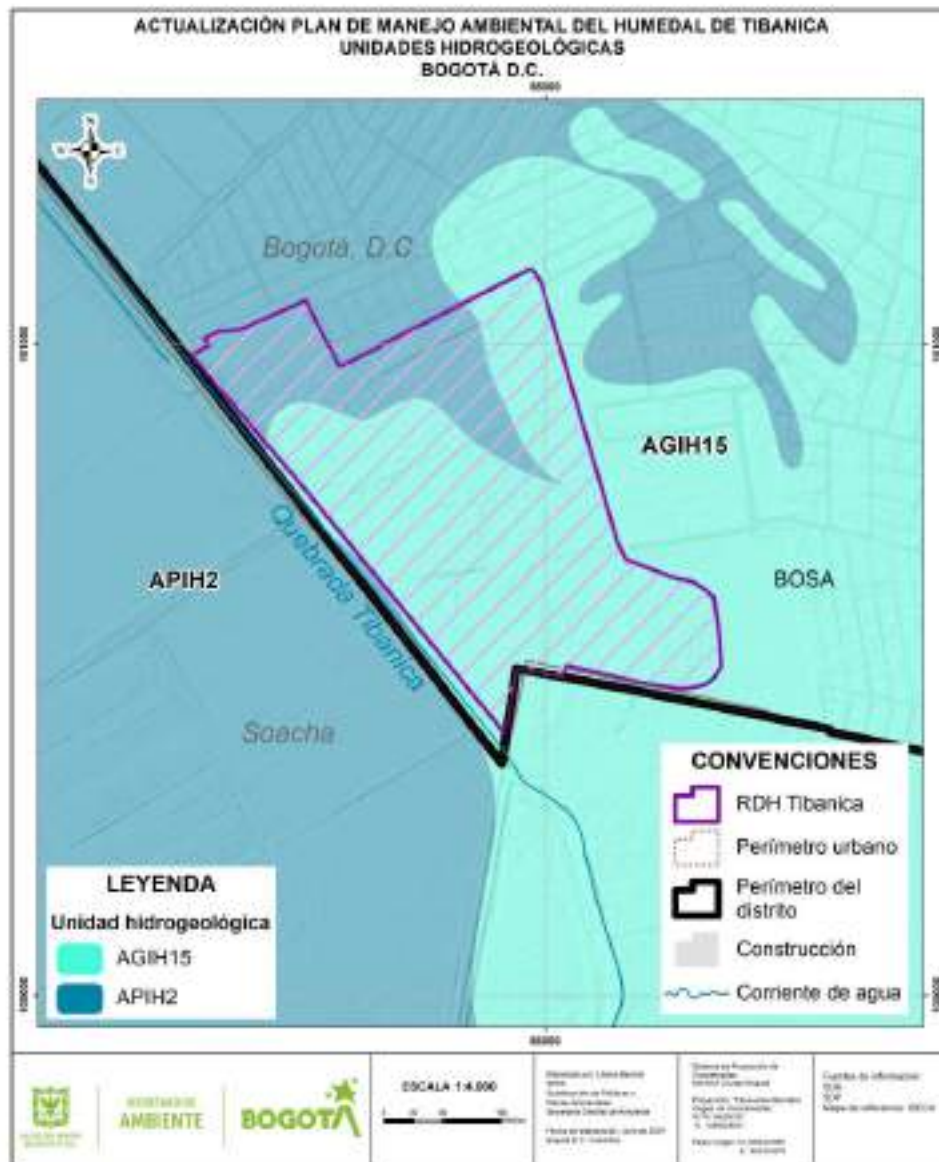
Figura 34. Unidades hidrogeológicas.
